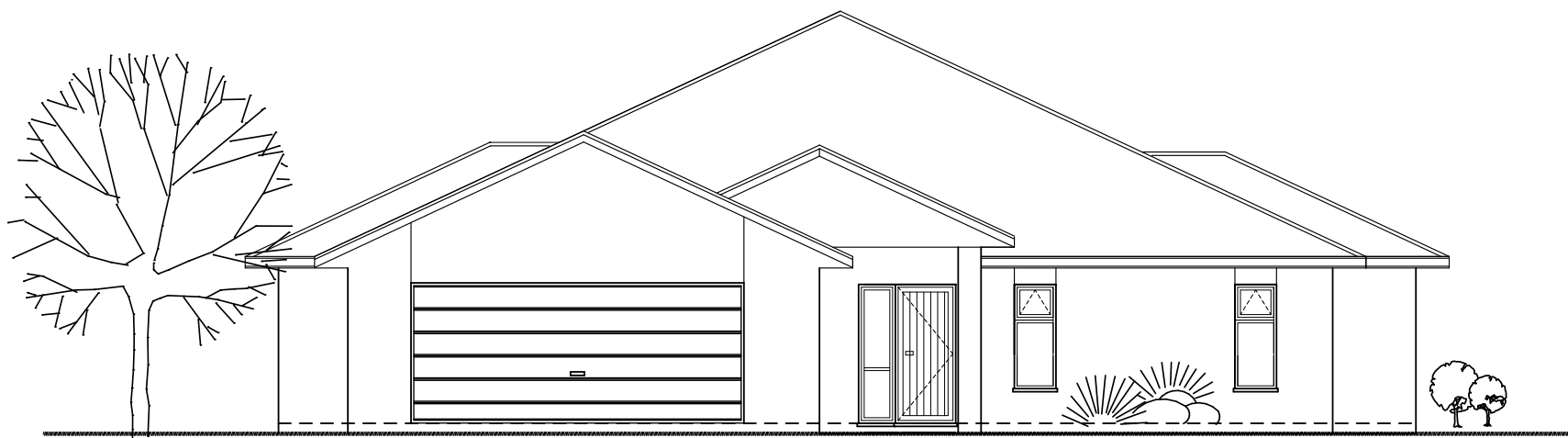
ELEVATION 1
