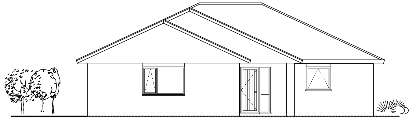
ELEVATION 1
